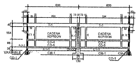
FACHADA ESTRUCTURAL POSTERIOR
