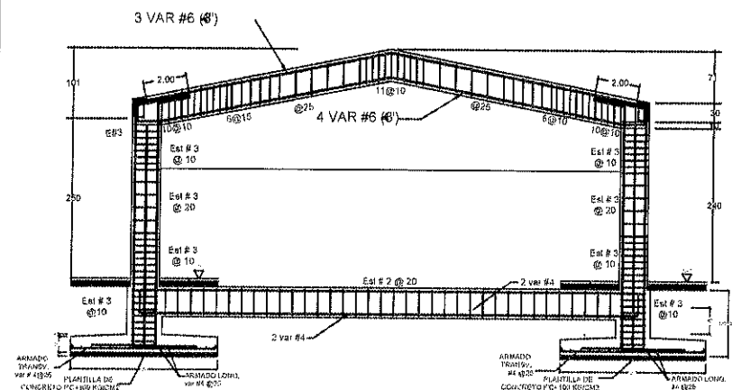
DETALLE DE MARCO ESTRUCTURAL
