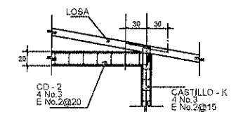
DETALLE - 4
