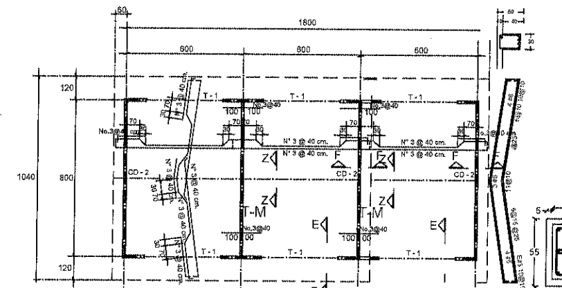
PLANTA ARMADO LOSA DE AZOTEA
