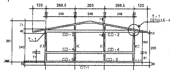
FACHADA ESTRUCTURAL MUROS CABECEROS
