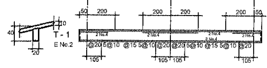
PLANTA ARMADO LOSA DE AZOTEA
