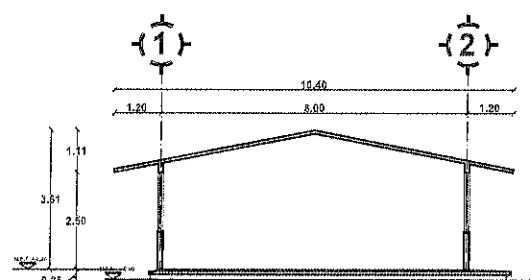
SECCIÓN Y-Y'
