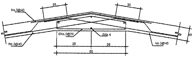
DETALLE DE CUMBRERA EN CUBIERTA CORTE Z - Z
