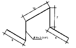
ISOMETRICO SILLETA
