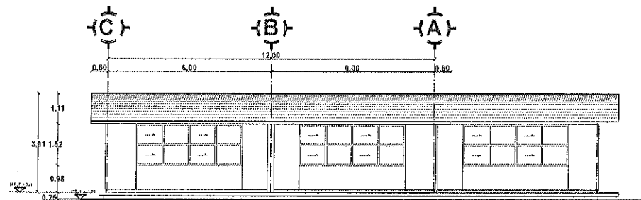
ALZADO POSTERIOR
