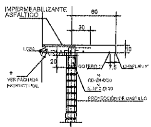
CORTE F - F
