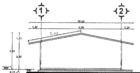
FACHADA LATERAL
