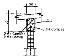
DETALLE - 3
