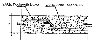
DETALLE DOBLEZ DE VARILLAS
