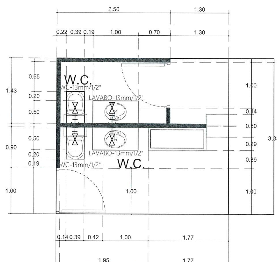
IH PLANTA HIDRUALICA BAÑOS 1/100
