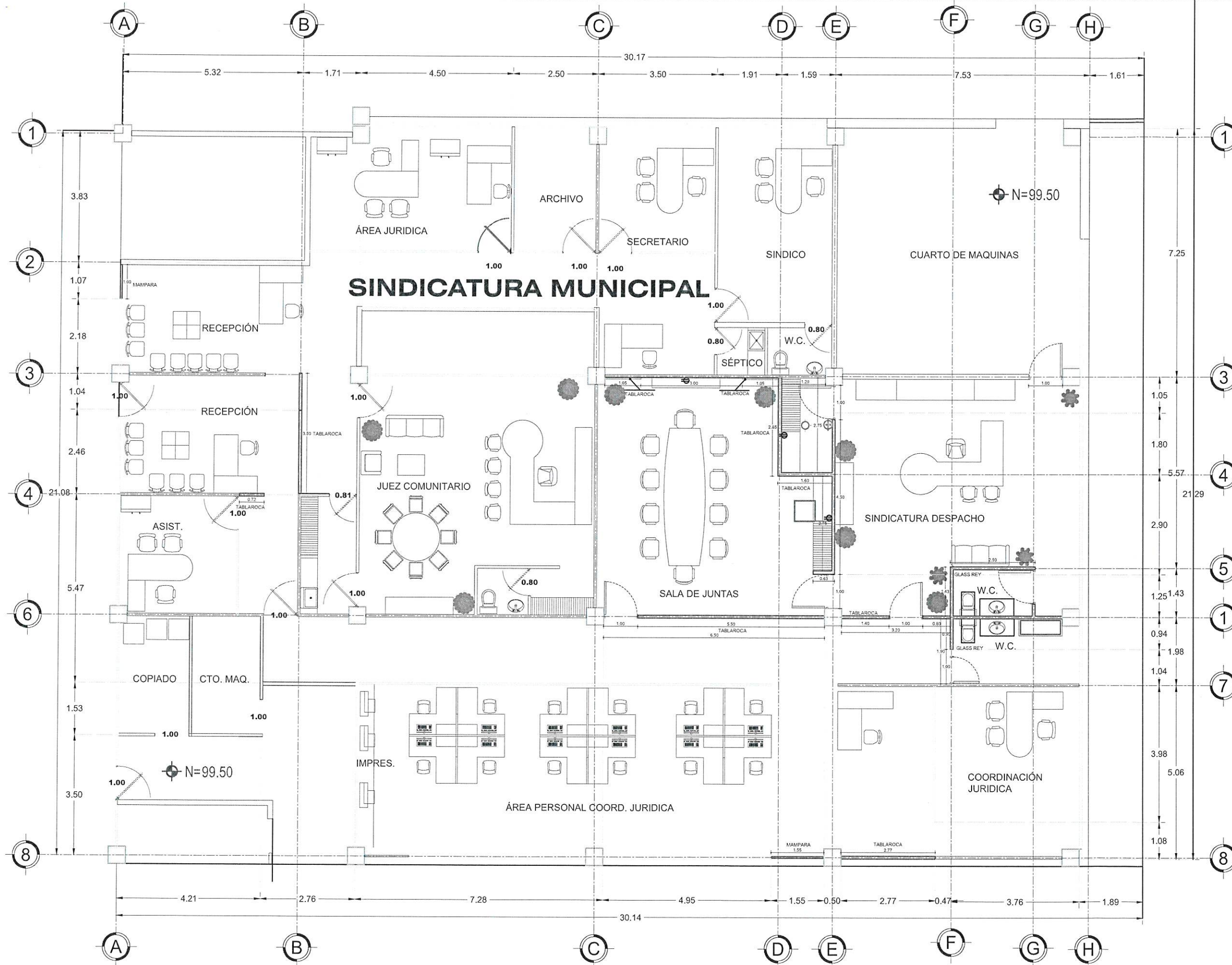
A PLANTA BAJA SINDICATURA 1/100
