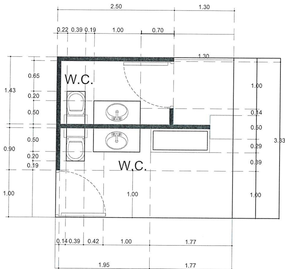
A PLANTA BAJA BAÑOS 1/100
