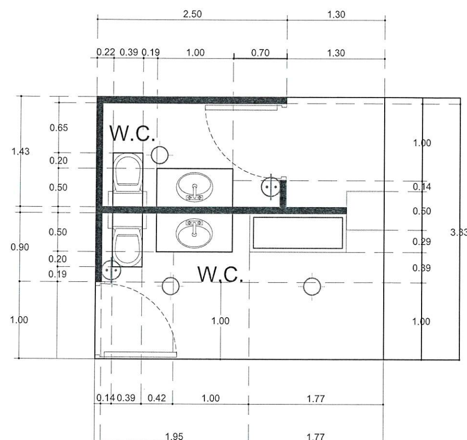
IE PLANTA ELECTRICA BAÑOS 1/100
