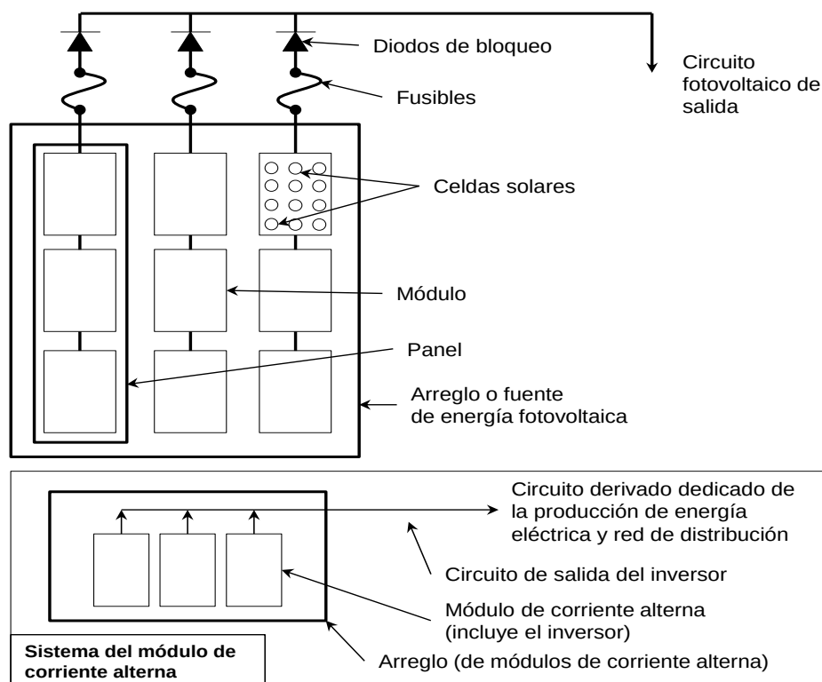
Figura 690-1(a) Identificación de los componentes de un sistema solar fotovoltaico
