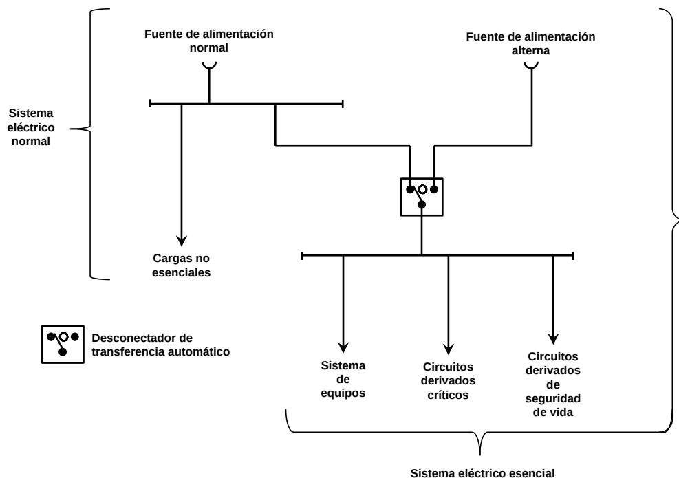
FIGURA 517-30 (b). - Requisito mínimo de un desconectador de transferencia para hospitales y establecimientos para la atención médica de pacientes ambulatorios, con una demanda máxima de hasta 150 kilovoltamperes de la carga conectada al sistema eléctrico esencial.
