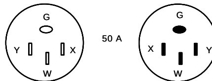
127/220 V, 50 A, 3 polos, 4 hilos, tipo de puesta a tierra
