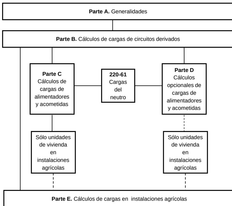
Figura 220-1 Métodos de cálculo para circuitos derivados, alimentadores y acometidas
