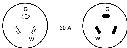
127/220 V, 30 A, 3 polos, 2 hilos, tipo de puesta a tierra
