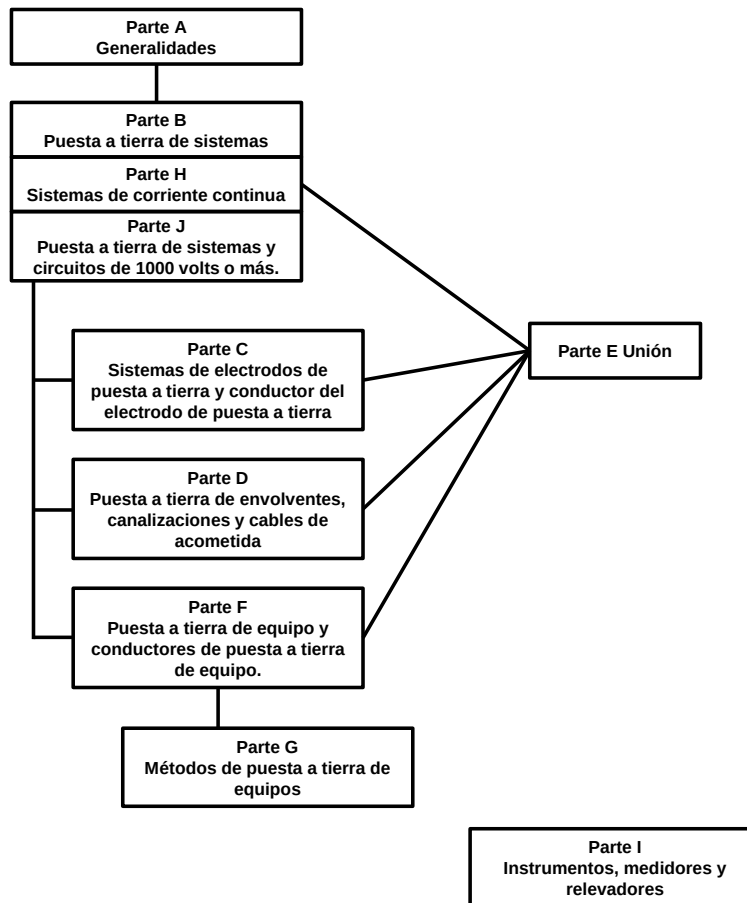
Figura 250-1 Puesta a tierra y unión.
