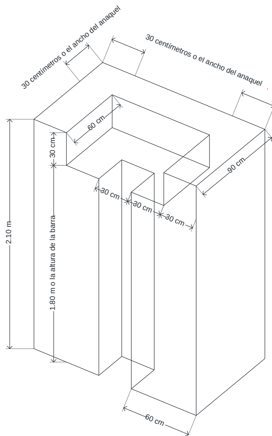
Figura 410-2 Espacio de almacenamiento del armario.
