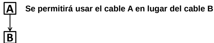
FIGURA 800-154.- Jerarquía de sustituciones de cables.
