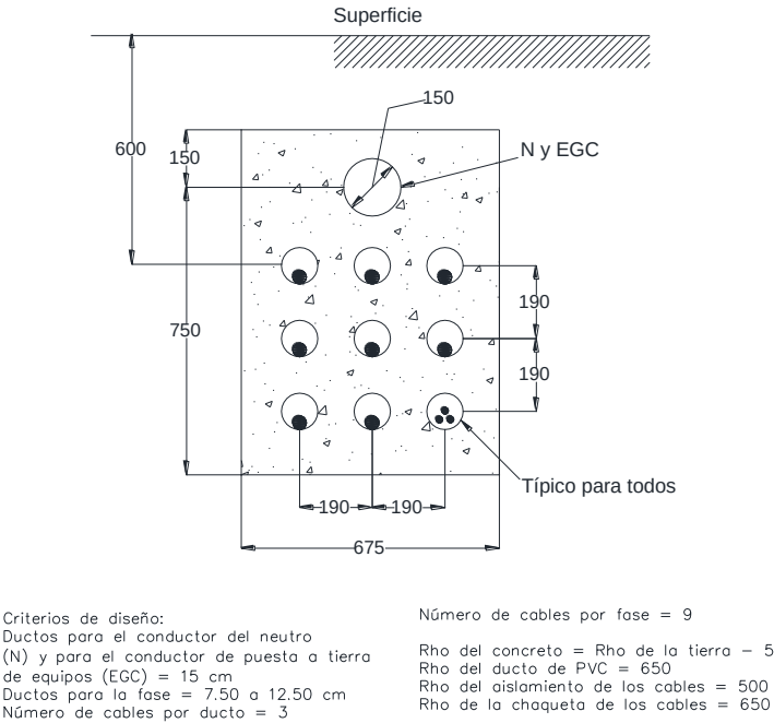
FIGURA B. 310-15(B)(2)(2) Dimensiones de la instalación de cables para usarlas con las Tablas B.310.15(B)(2)(5) hasta la Tabla B.310.15(B)(2)(10)
