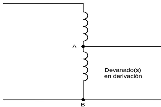
Figura 450-4 Autotransformador
