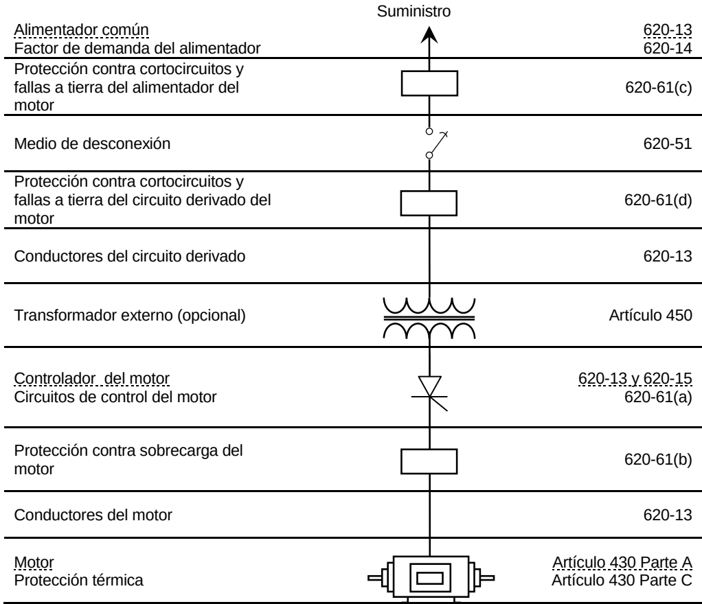
Figura 620-13 Diagrama unifilar
