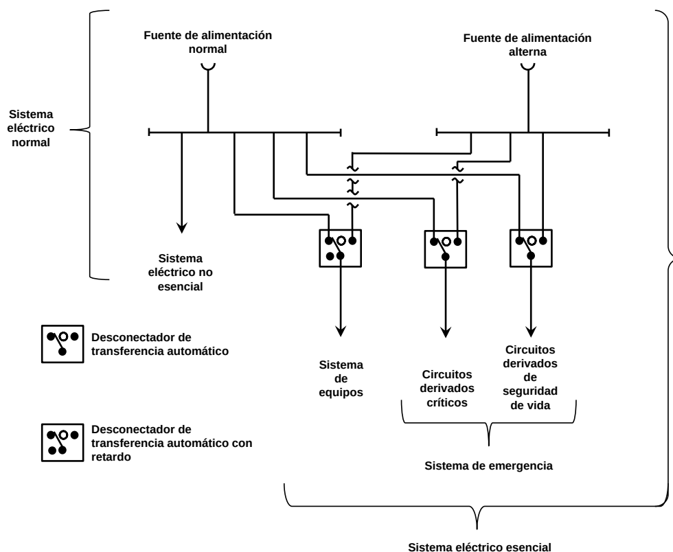
FIGURA 517-30 (a). - Requisito mínimo de tres desconectadores de transferencia automáticos para hospitales y establecimientos para la atención médica de pacientes ambulatorios, con una demanda máxima superior a 150 kilovoltamperes de la carga conectada a los dos sistemas el de emergencia y el de equipos.
