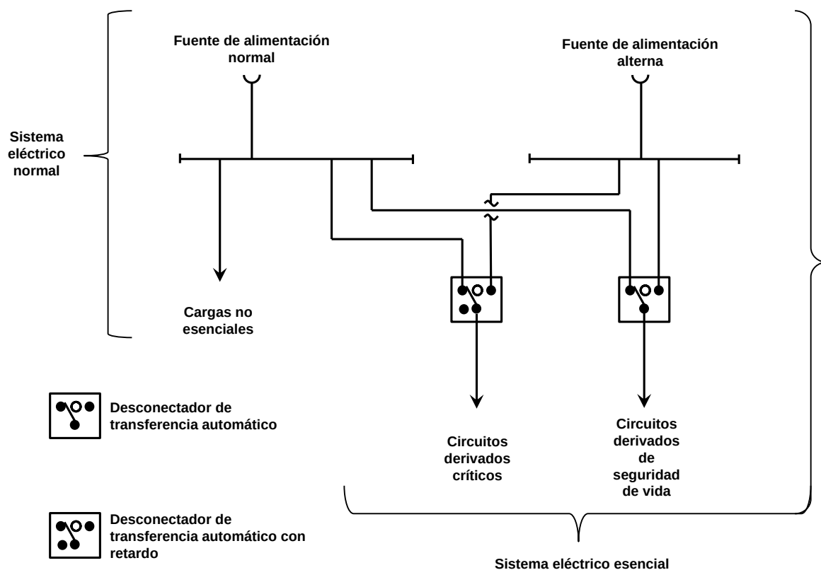
FIGURA 517-41 (a). - Arreglo de dos desconectores de transferencia para áreas de atención limitada.
