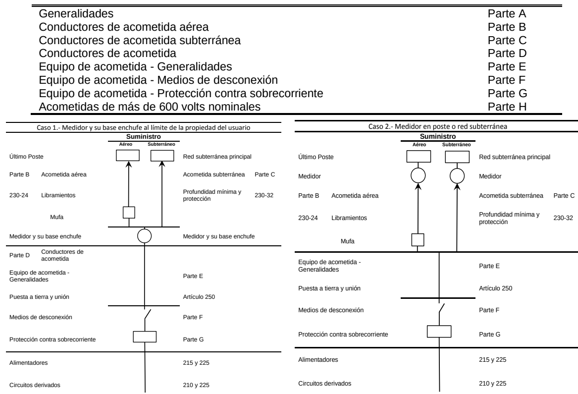
FIGURA 230-1.- Acometidas
