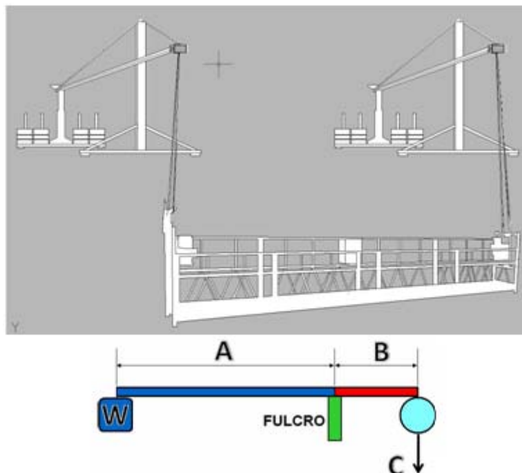
Figura 7 Contrapesos en andamios suspendidos
